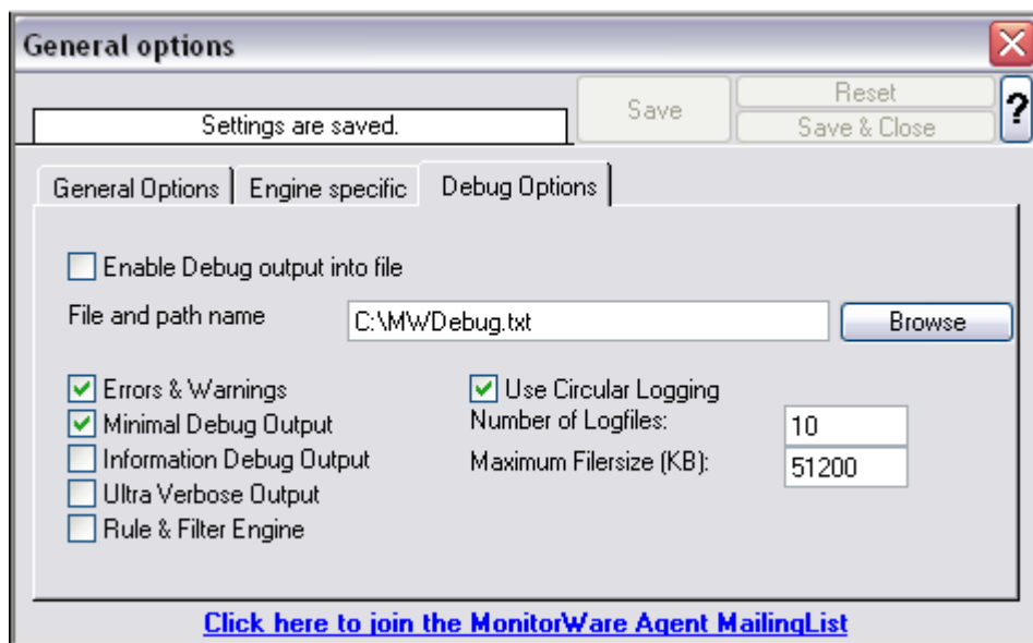
Figure3: Debug Options
