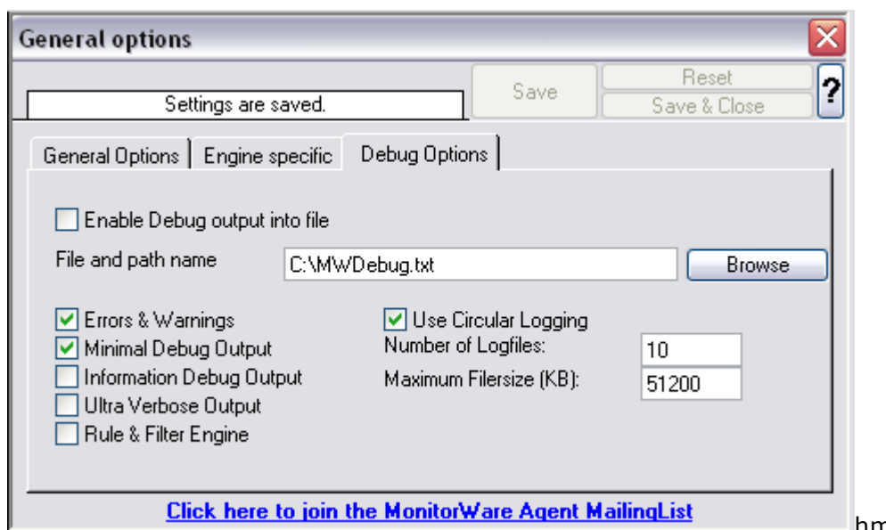
Figure3: Debug Options
