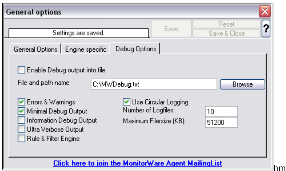
Figure3: Debug Options
