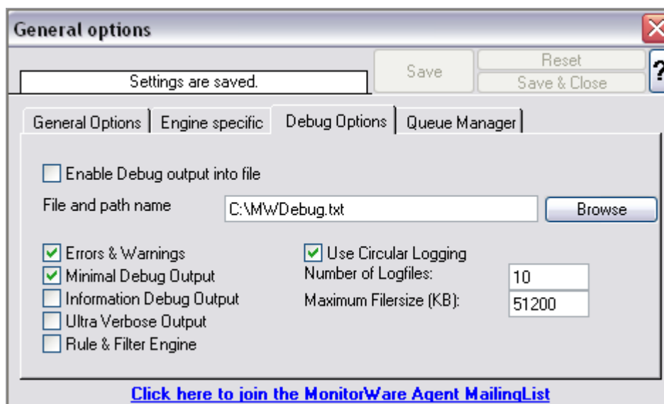
Figure3: Debug Options
