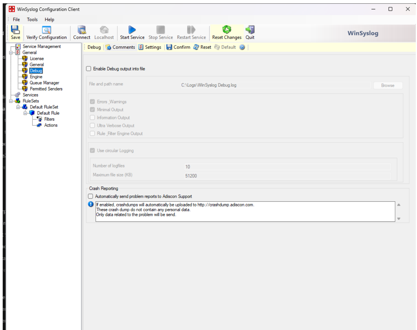
WinSyslog Debug options
